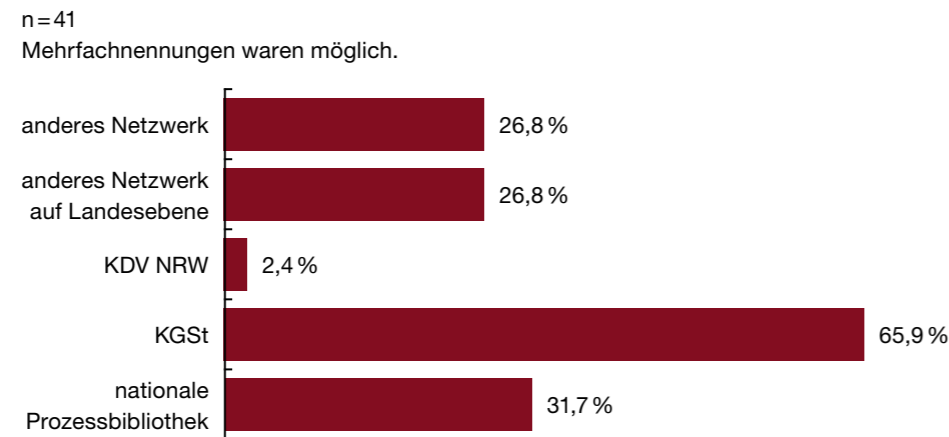
Abb. 30 Relevante Netzwerke
