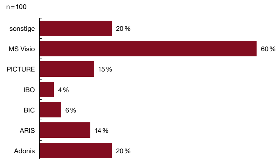
Abb. 16 Genutzte Tools
