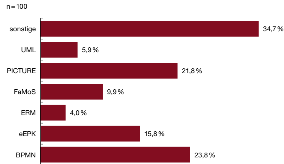
Abb. 15 Genutzte Notationen
