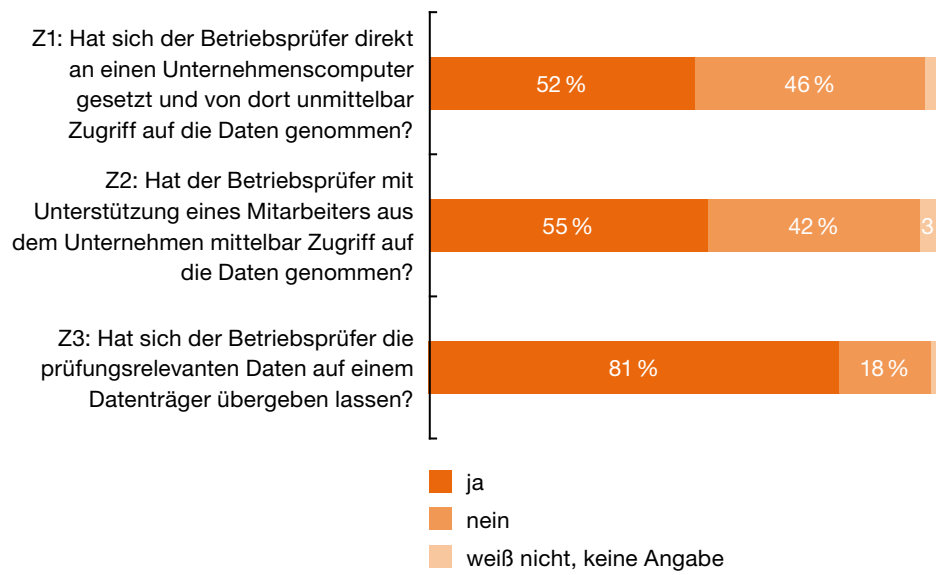
Abb. 16 Genutzte Zugriffsarten
